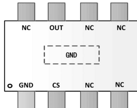
ESOP 8
