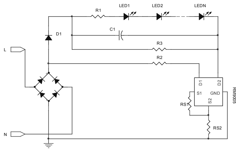
图 1: 典型驱动方案
