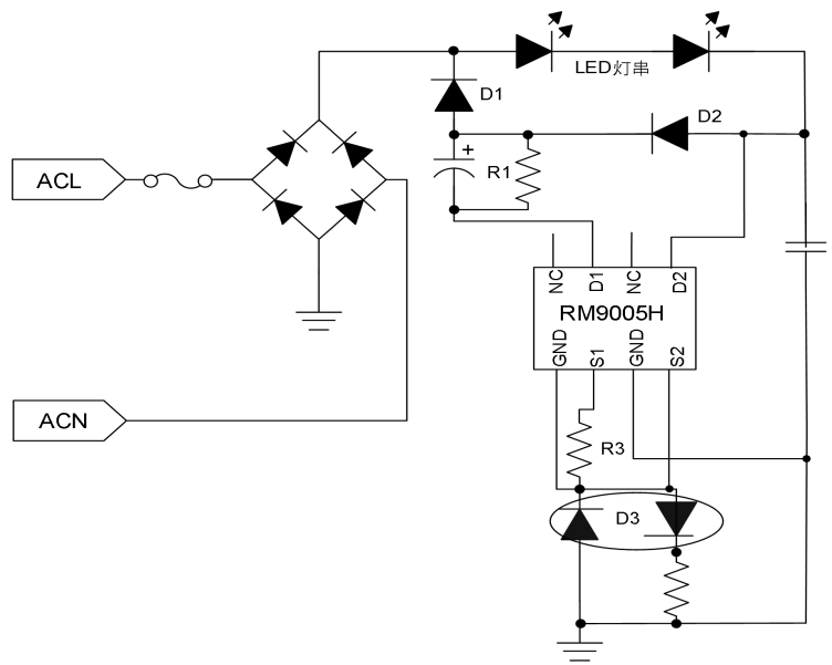
图 2: 半压应用典型方案
