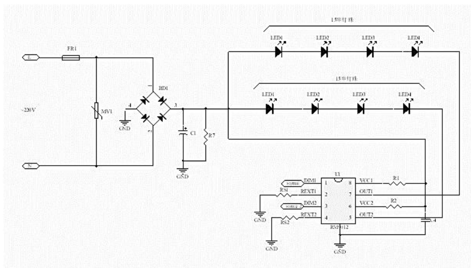
图 1:典型电路
