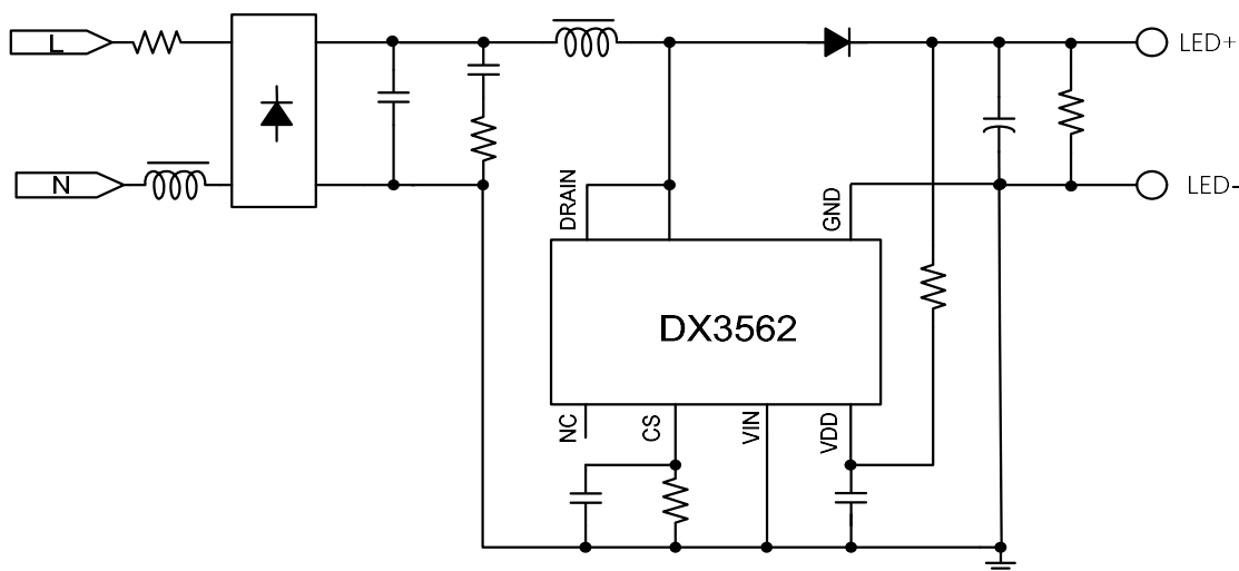
图 6: DX3562 BOOST 结构
