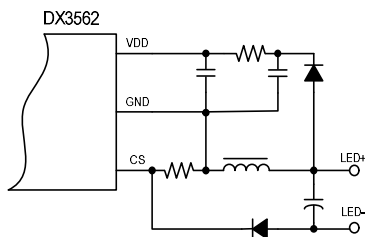
图 1:浮地结构 VDD 供电
