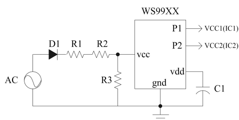
图1 供电示意图
