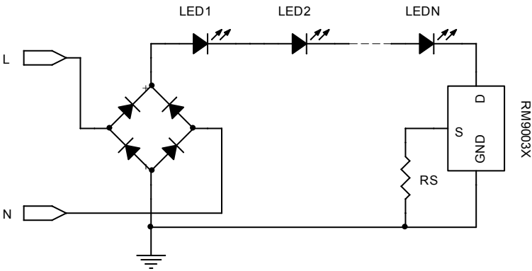
图 1:单个驱动
