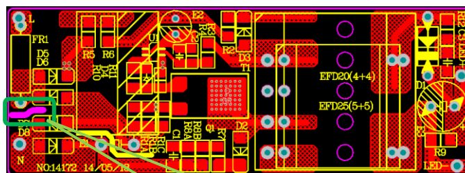
开槽增加安全距离
