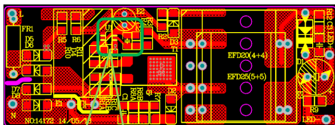
反馈元件的地紧挨 IC 地
