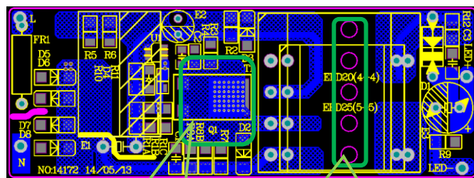
铜箔底部露铜
