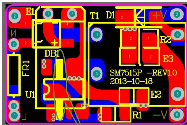
铺铜散热
