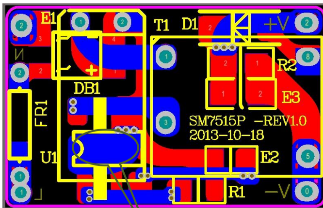
铺铜散热
