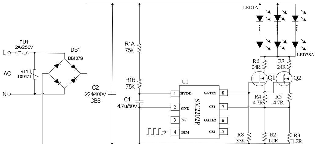
图 6 SM2202P 50W 低 PF 无频闪应用方案原理图
