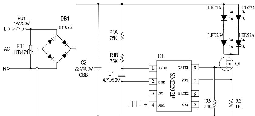
图4 SM2202P 36W 高 PF 三段调色应用方案原理图
