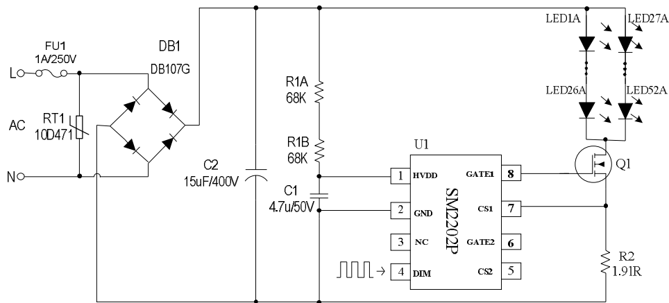
图 5 SM2202P 30W 低 PF 无频闪三段调色应用方案原理图
