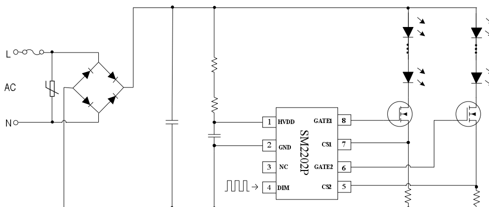
图3 SM2202P 方案应用示原理图
