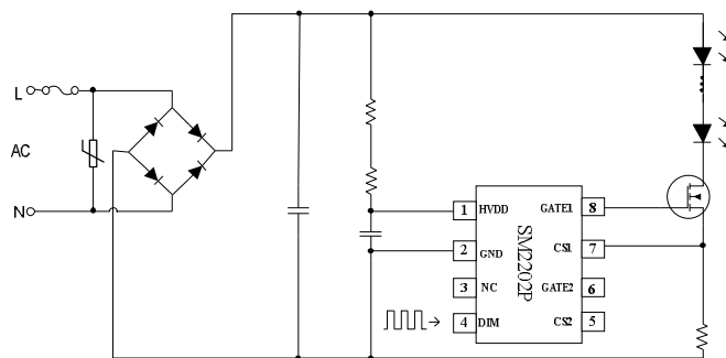
图 2 SM2202P 单通道（二选一）典型应用示意图
