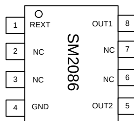
ESOP8
