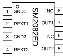
ESOP8
