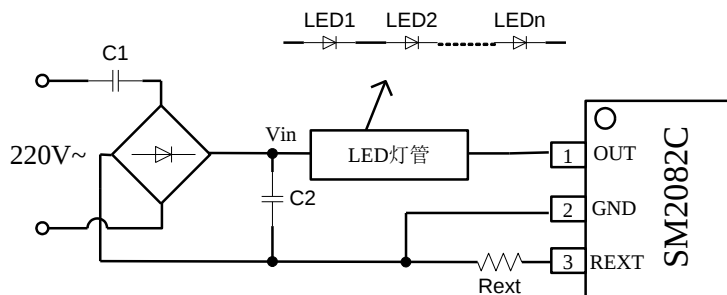
图 5 SM2082C 典型应用电路—交流电源输入
