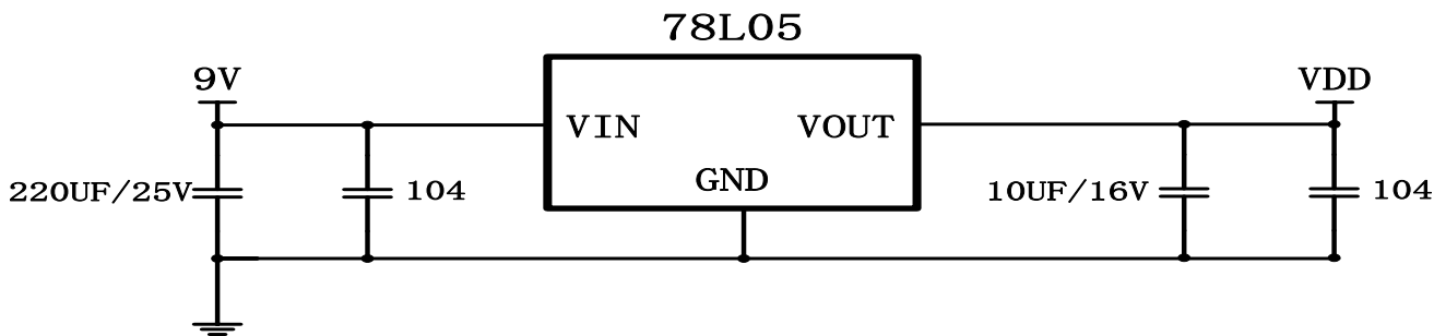
电源电路
