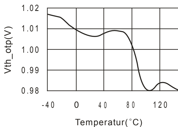
Vth_otp(V) vs Temperatur(°C)
