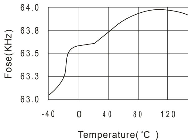
Fose(KHz) vs Temperature (°C )
